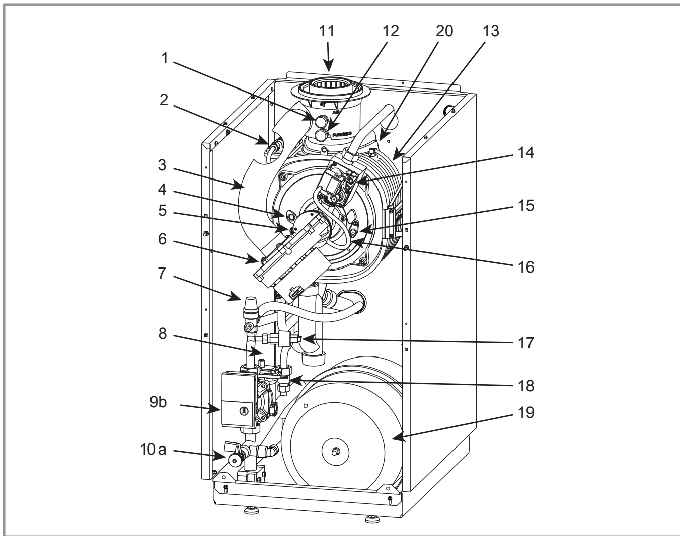
figure 9 - Organes de l'appareil (perfinox condens)
