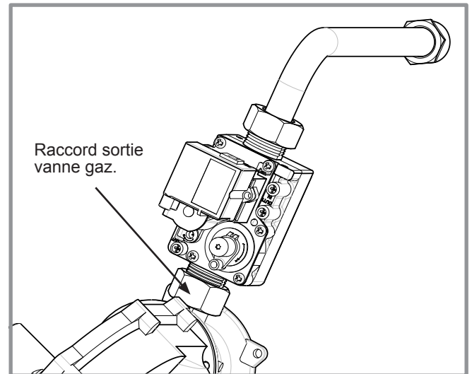
figure 22 - Accès au diaphragme
