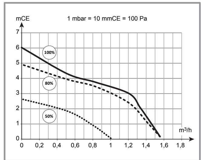
figure 6 - Pressions et débits disponibles perfinox condens duo 5028
