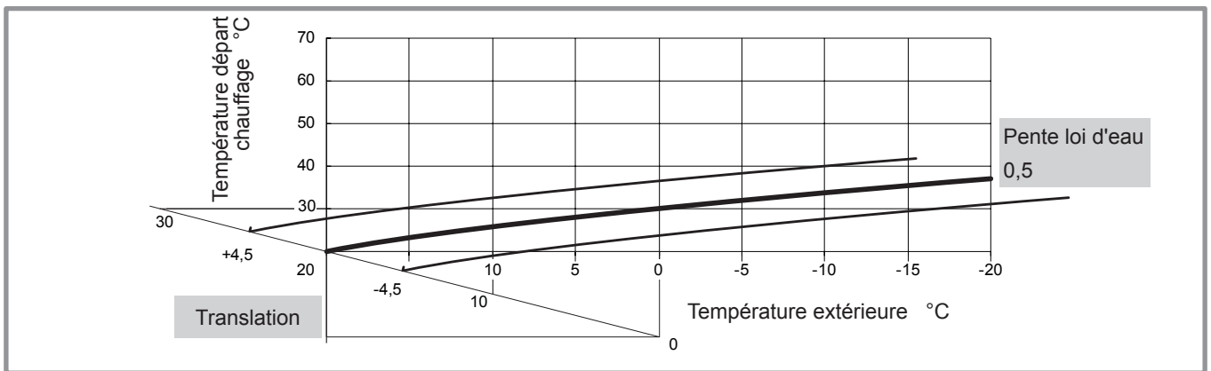
figure 40 - Translation de la courbe de chauffe (ligne 76)
