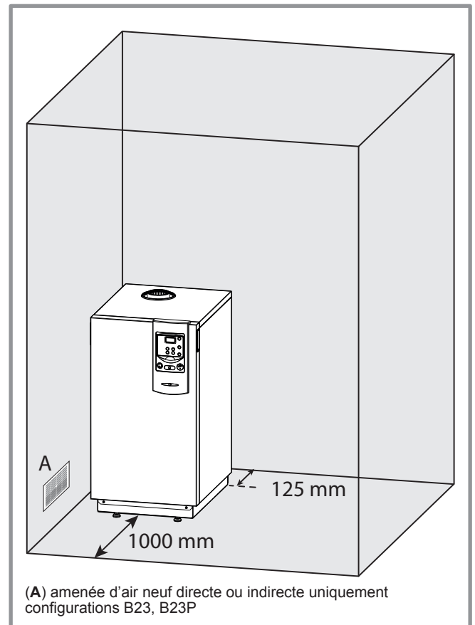
figure 13 - Dégagements minimum d'installation autour de la chaudière
