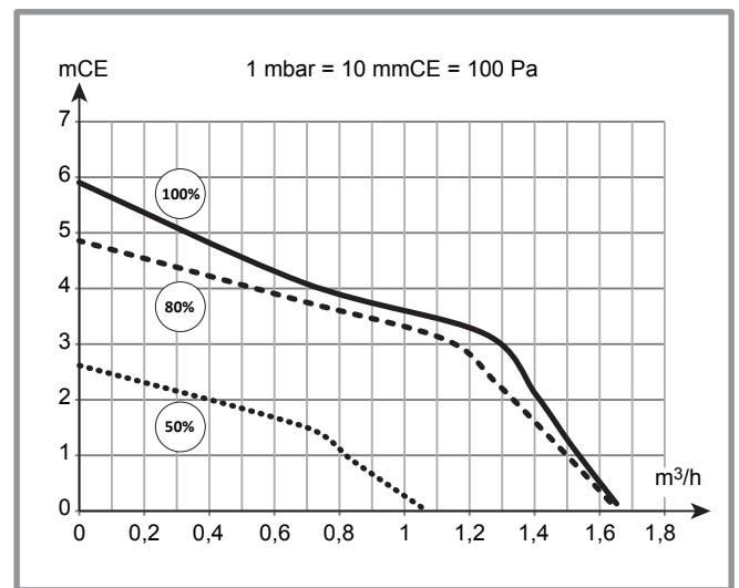
figure 5 - Pressions et débits disponibles perfinox condens duo 5024
