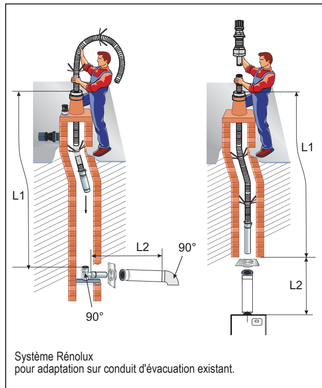
figure 17 - Possibilités de raccordement (type C13 et C33)
