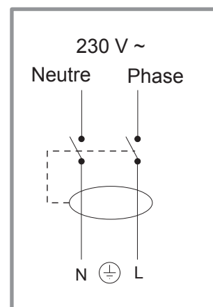
figure 26 - Protection différentielle
