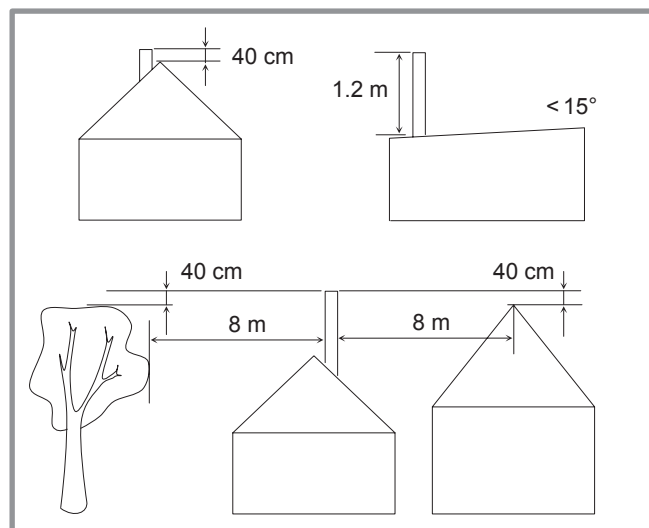
figure 16 - Hauteur de la souche du conduit d'évacuation (B23, B23p)
