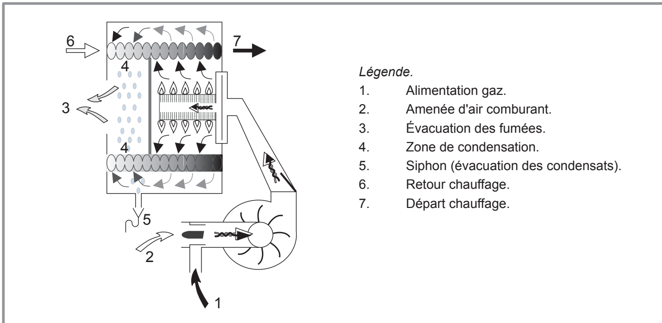
figure 6 - Principe brûleur et échangeur condenseur
