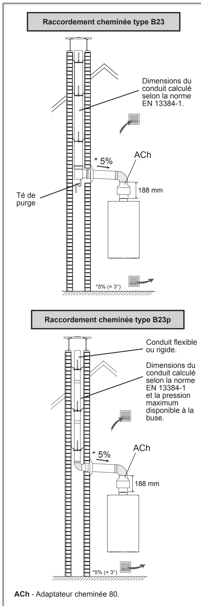
figure 17 - Possibilités de raccordement (type B23 et B23p)
