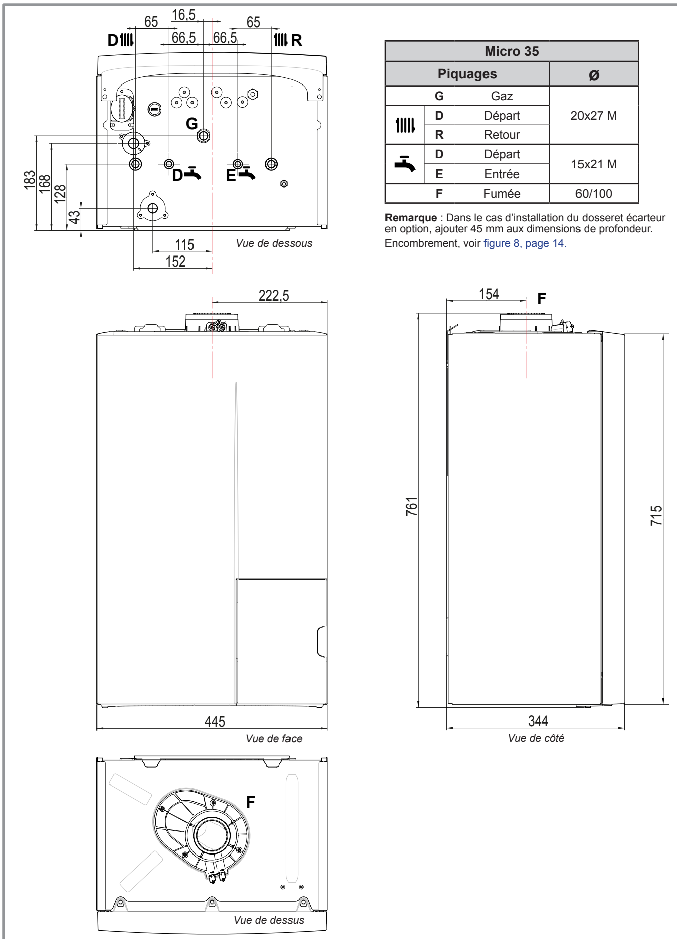
figure 4 - Micro 35 - Largeur 445 (dimensions en mm)
