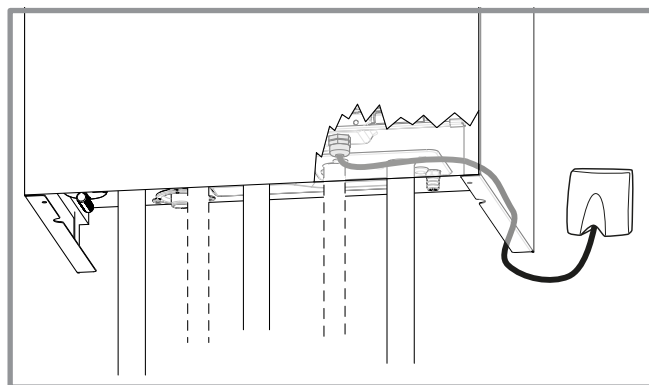
figure 19 - Alimentation électrique 230 V (50 Hz)
