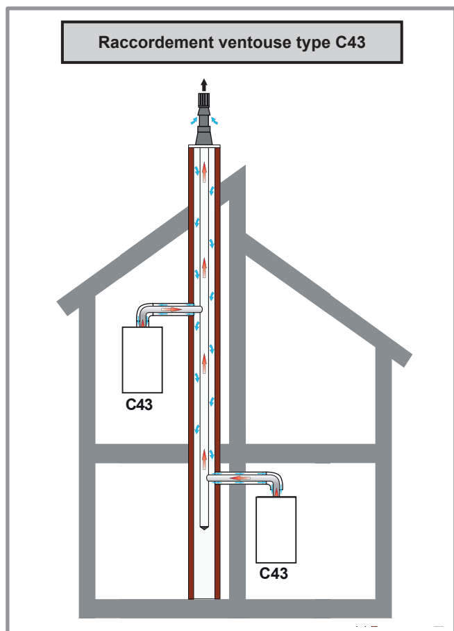
figure 15 - Possibilités de raccordement (type C43)
