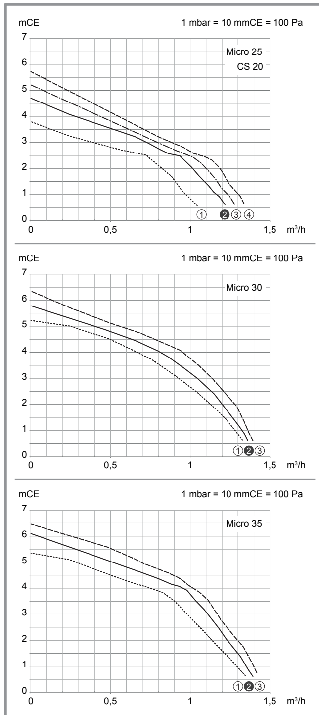
figure 25 - Pressions et débits hydrauliques disponibles
