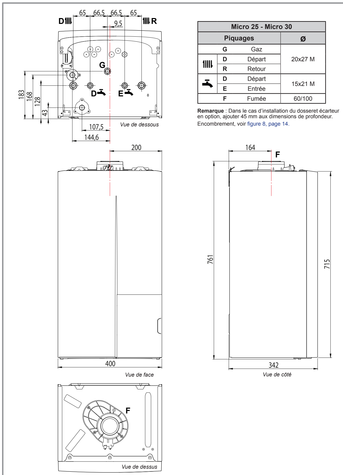
figure 3 - Micro 25 - Micro 30 - Largeur 400 (dimensions en mm)
