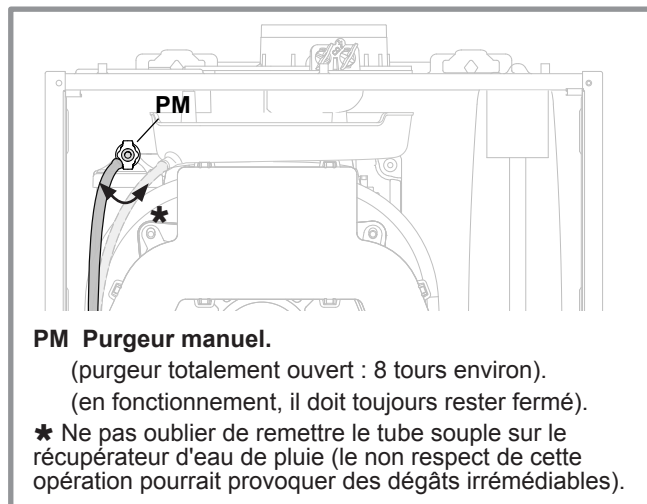
figure 32 - Rappel : tube souple en place
