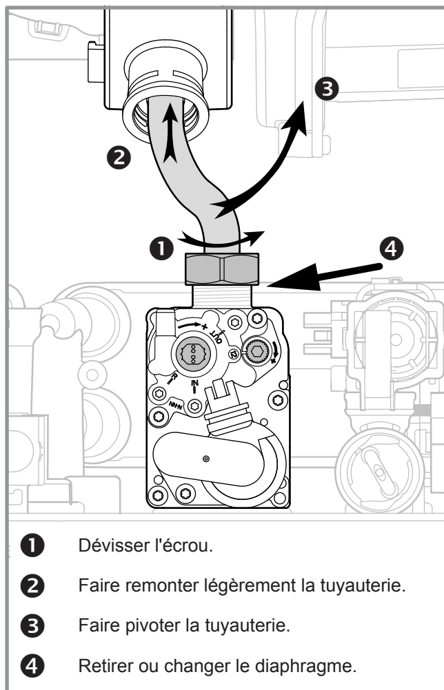
figure 11 - Accès au diaphragme
