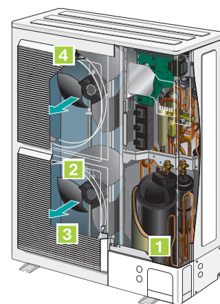
Unité extérieure
